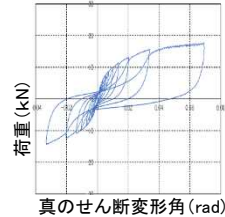
荷重と真のせん断変形角との関係
